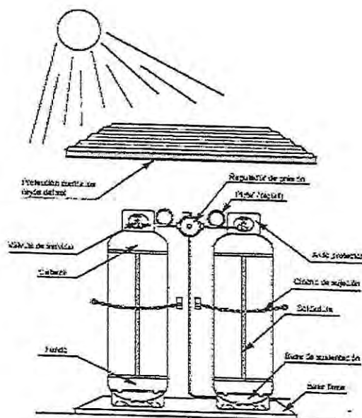
Figura 1. Instalación típica para cilindros portátiles.
