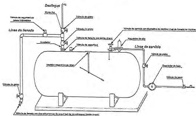
Figura 2. Instalación típica para tanques estacionarios
