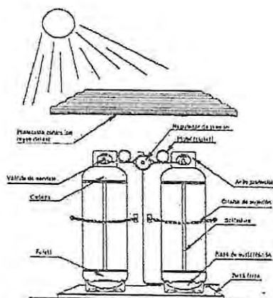
Figura 1. Instalación típica para cilindros portátiles.
