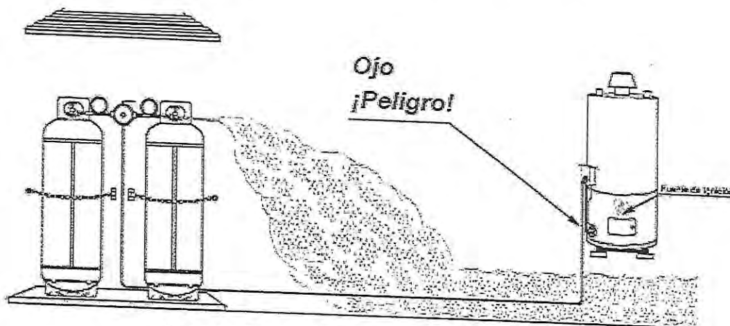
Figura 4. – Desplazamiento típico de una fuga de gas licuado
