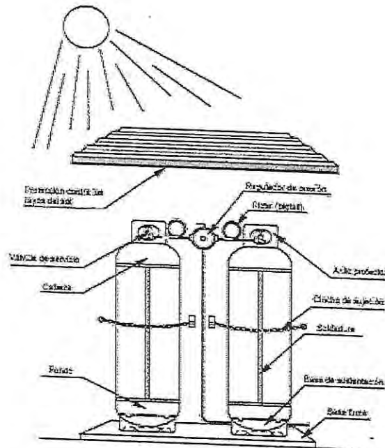
Figura 1. Instalación típica para cilindros portátiles.
