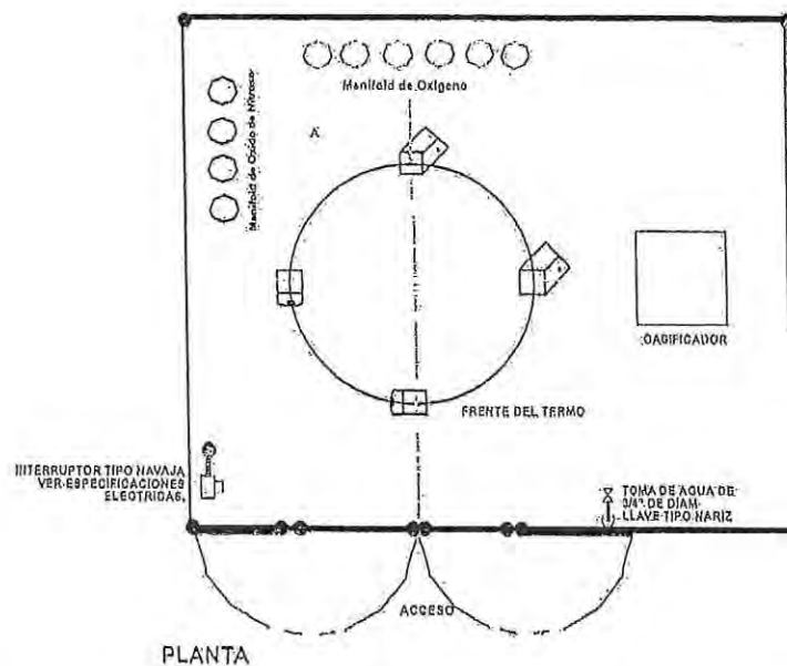
Figura 10.6.1.4 Ilustra vista en planta control de gases con manifold con suministro principal con termo estacionario y respaldo con cilindros de alta presión.
