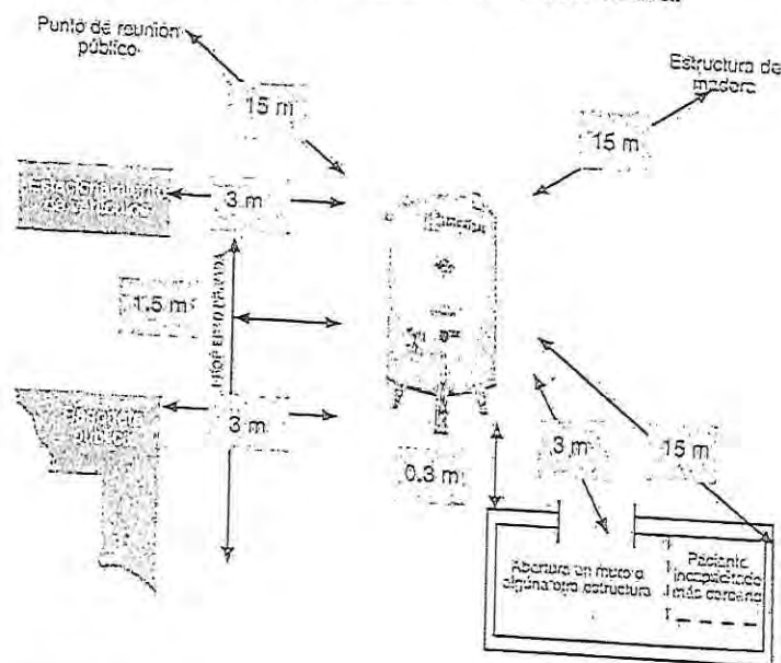
Figura 10.6.3.1 Ilustra las distancias mínimas de seguridad para la instalación de la central de gases.
