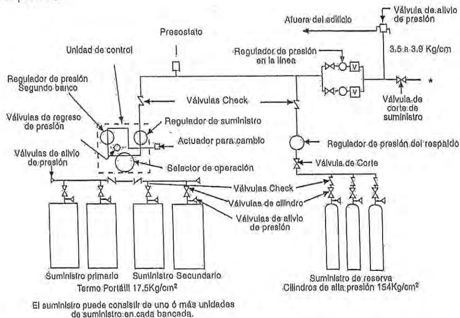
Figura 10.4.1 Diagrama de un manifold para oxígeno con suministro de termos portátiles y reserva de cilindros.
