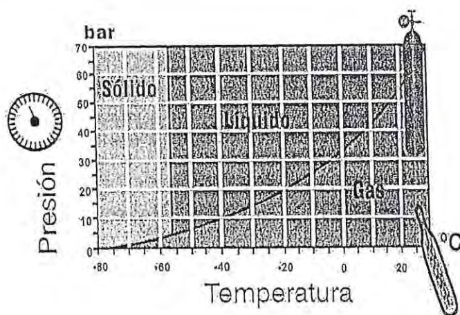
Figura 12.2.1 Estados físicos del Bióxido de Carbono.
