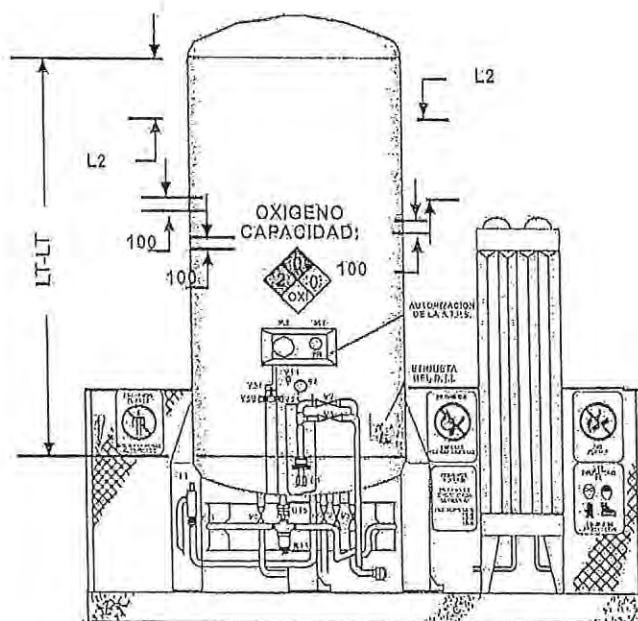
Figura 10.6.1.3 Ilustra Elevación de control de gases con manifold con suministro principal con termo estacionario y respaldo con cilindros de alta presión.
