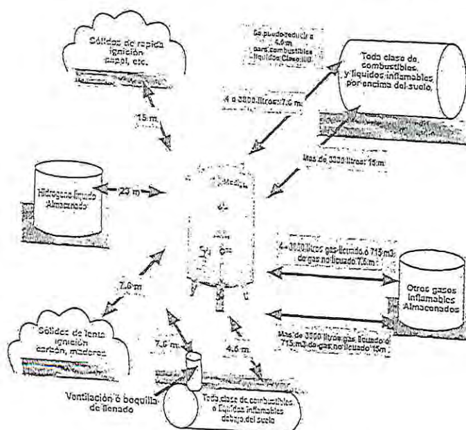
Figura 10.6.3.2 Ilustra los tipos de factores que establecen la situación de la central de gases.
