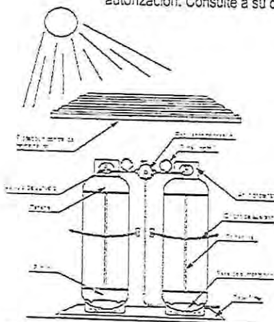
Figura 1. Instalación típica para cilindros portátiles
