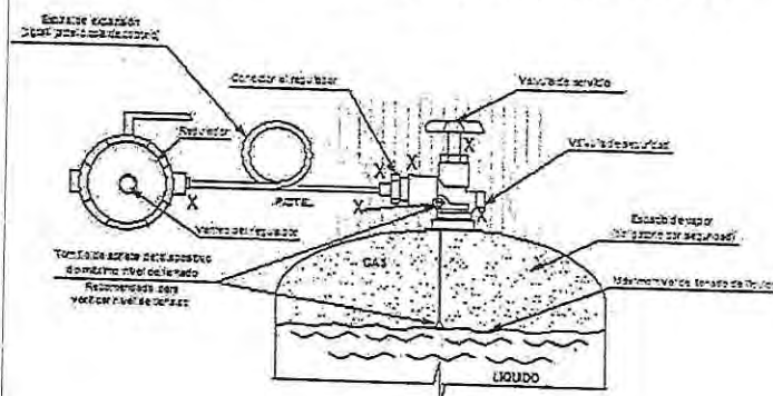
Figura 3. Muestra el dispositivo indicador de máximo nivel de llenado de líquidos, la espiral de expansión (píctel) y la localización de posibles puntos de fuga (X).
