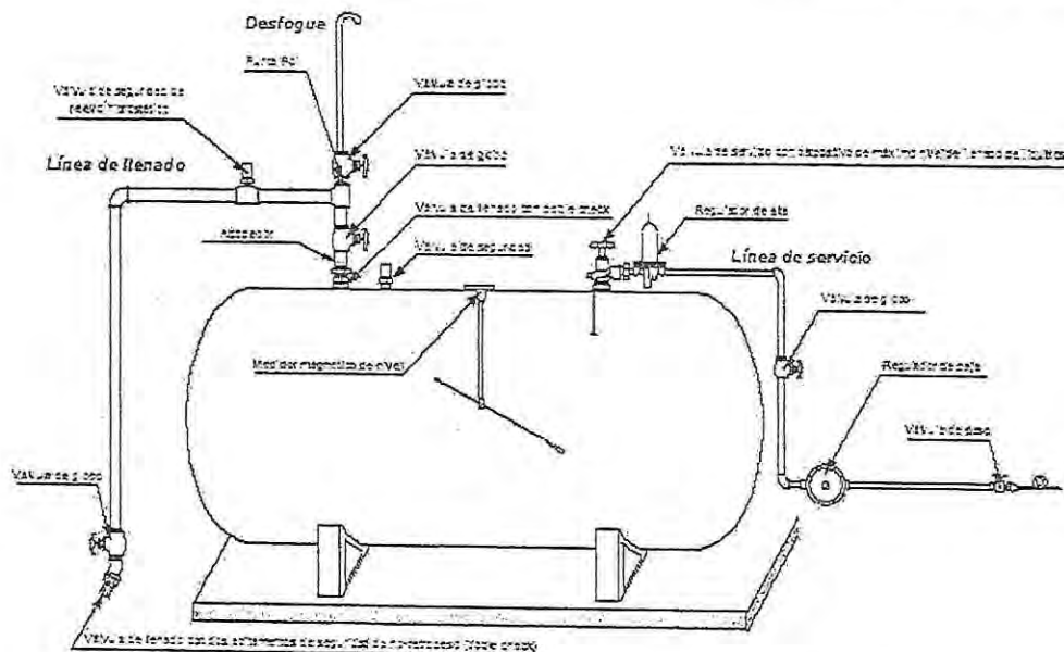
Figura 2. Instalación típica para tanques estacionarios
