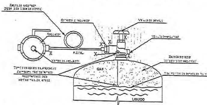
Figura 3. Muestra el dispositivo indicador de máximo nivel de llenado de líquidos, la espiral de expansión (pictel) y la localización de posibles puntos de fuga (X).
