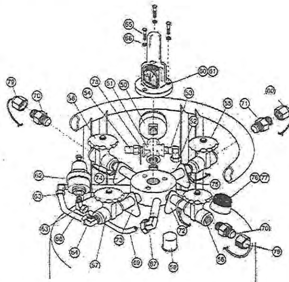
Figura. Componentes de la parte superior del termo portátil.
