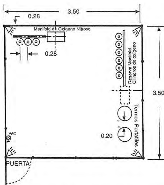
Figura 10.4.2 Plano de una central de gases para suministro de oxígeno con termos portátiles y respaldo de cilindros, y óxido nitroso con suministro y reserva de cilindros.
