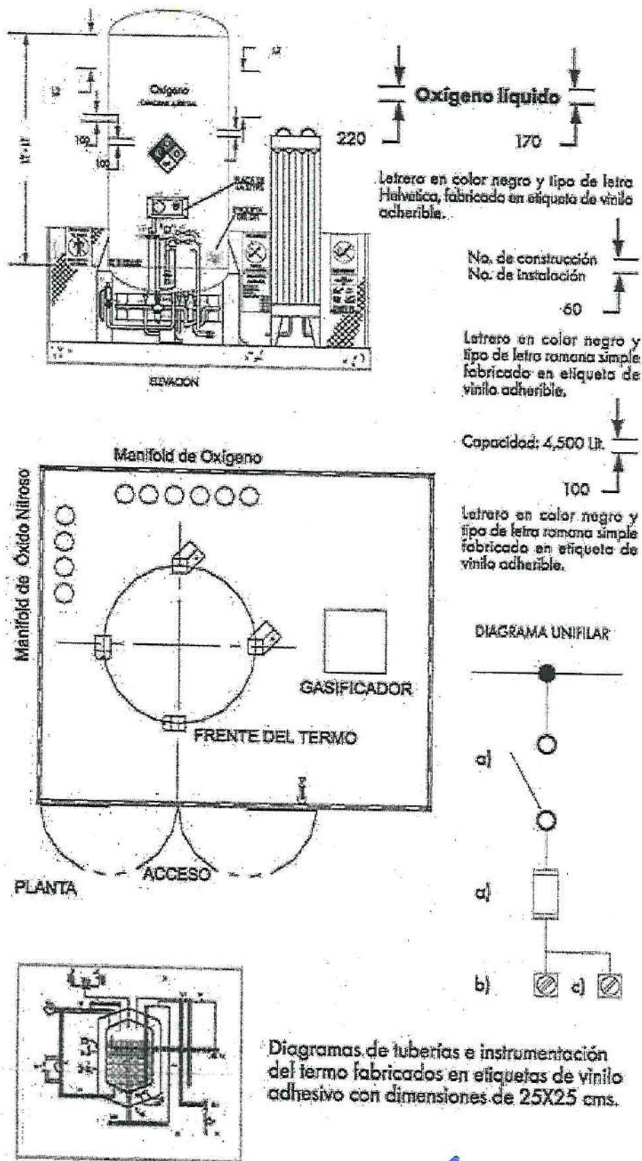
Figura 10.6.1.2 Ilustra central de gases con manifold con suministro principal con termo estacionario y respaldo con cilindros de alta presión.
