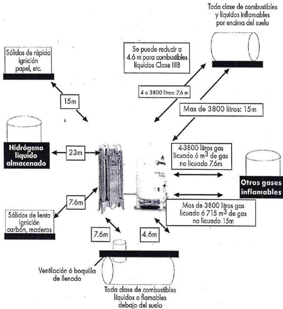
Figura 10.6.3.2 Ilustra los tipos de factores que establecen la situación de la central de gases
