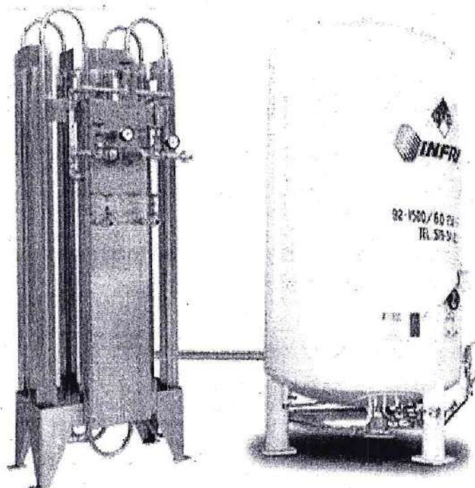
Figura 10.6.3 Ilustra el evaporador ambiental, transforma el oxígeno líquido a oxígeno gaseoso.
