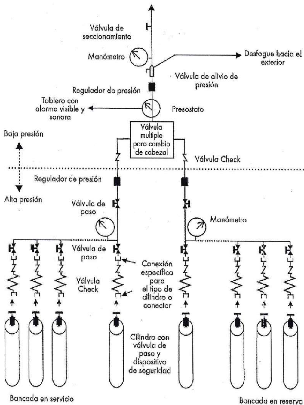
Figura 8.1.4.1 Esquema de un "manifold" para oxígeno
