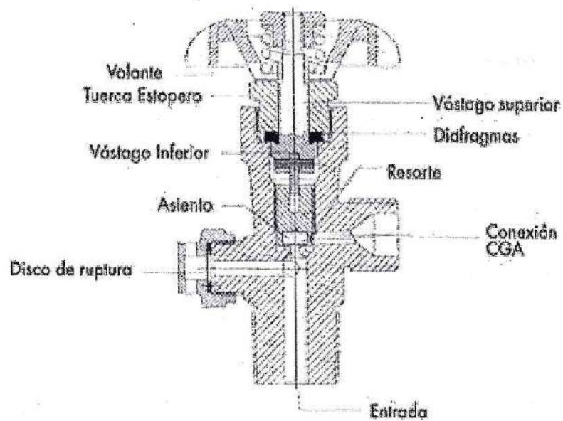
Válvula con sello de diafragma
