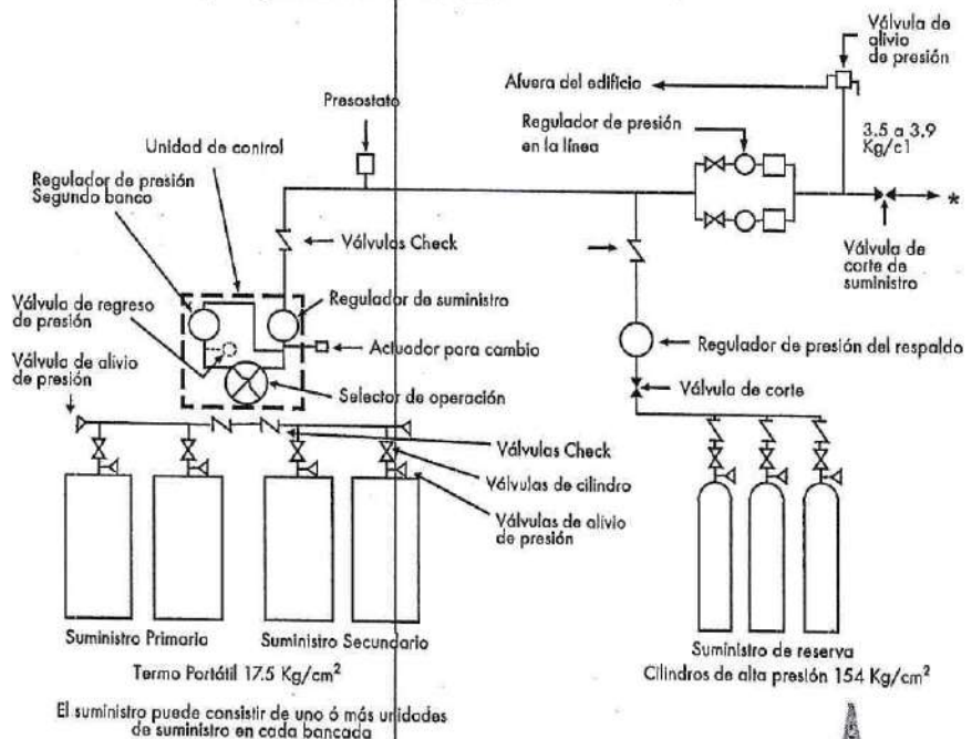
Diagrama de un manifold para oxígeno con suministro de termos portátiles y reserva de cilindros.
