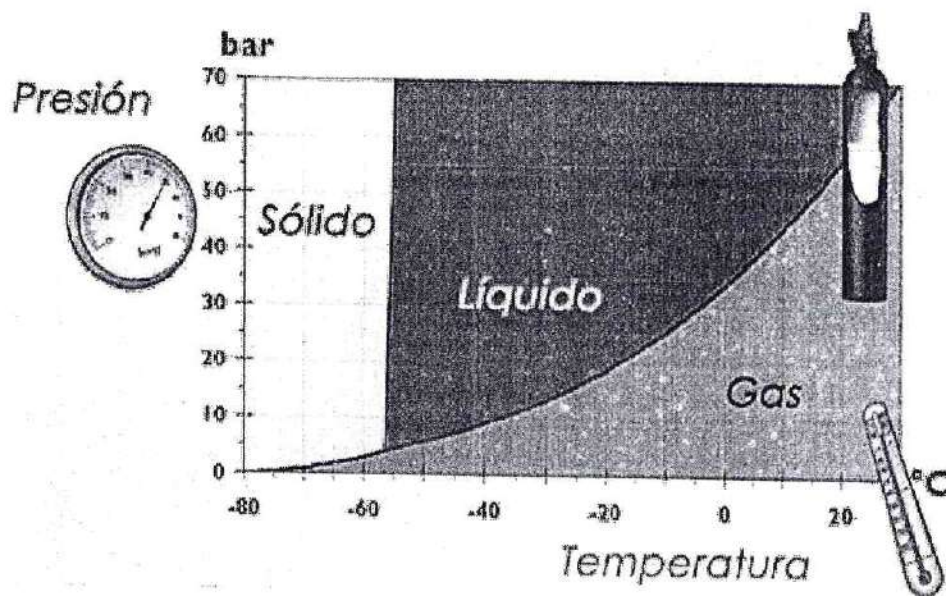
Figura 12.2.1 Estados físicos del Bióxido de Carbono.
