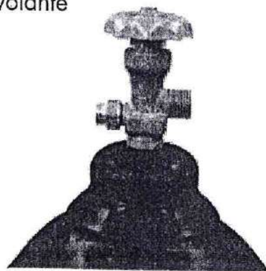
Figura 8.2.3.2 Ilustra la válvula tipo volante
