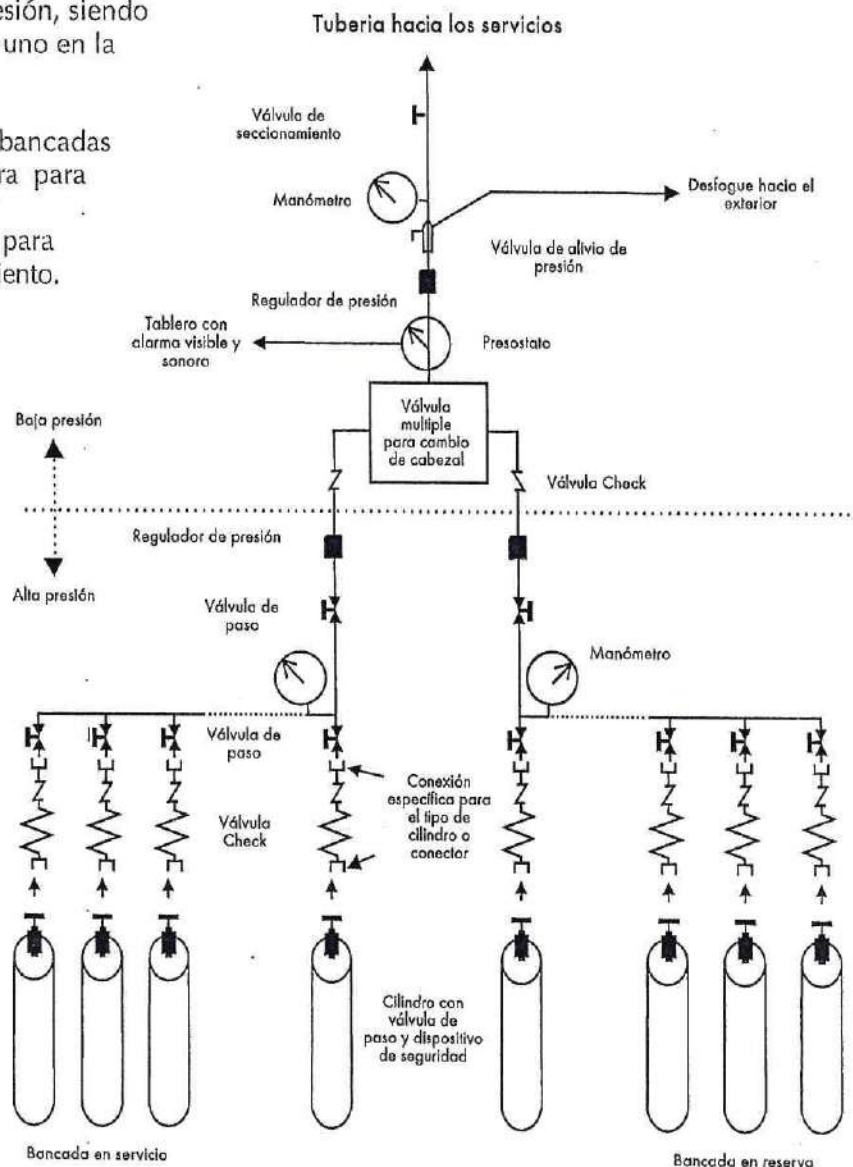
Esquema de un "manifold" para oxígeno.
