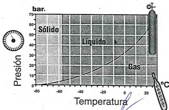
Figura 12.2.1 Estados físicos del Bióxido de Carbono.
