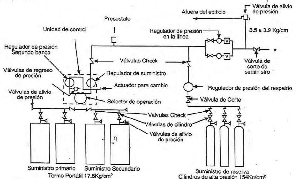
Figura 10.4.1 Diagrama de un manifold para oxígeno con suministro de termos portátiles y reserva de cilindros.
