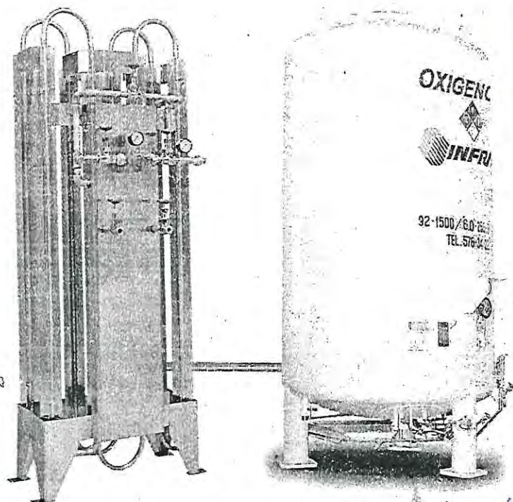
Termo estacionario con su evaporador.
