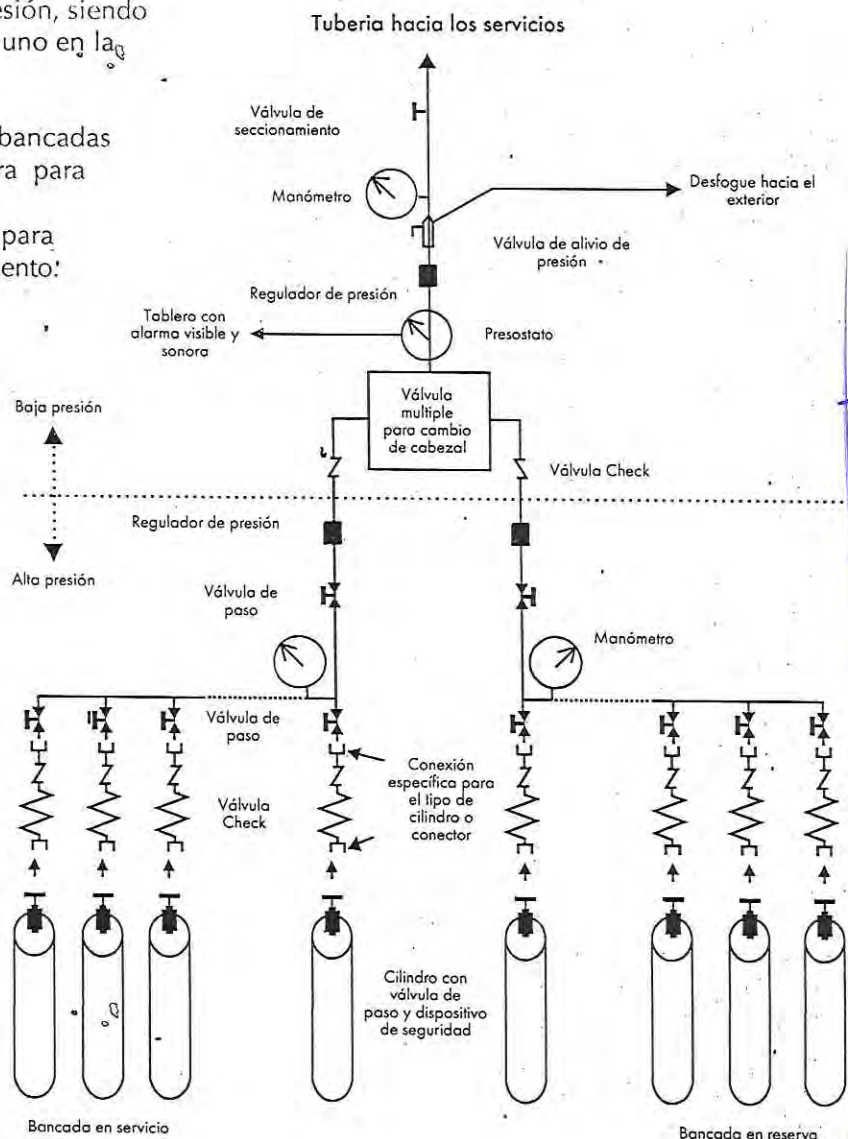
Esquema de un "manifold" para oxígeno.
